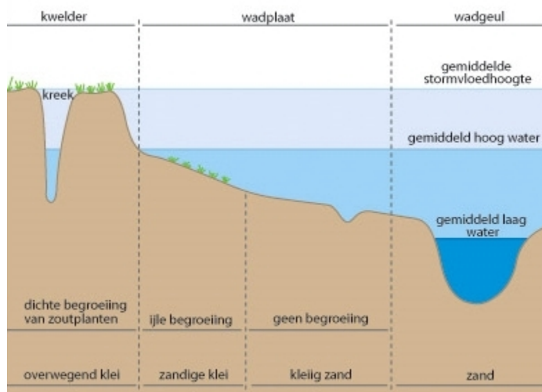
DWARSDOORSNEDE WADDENGEBIED
